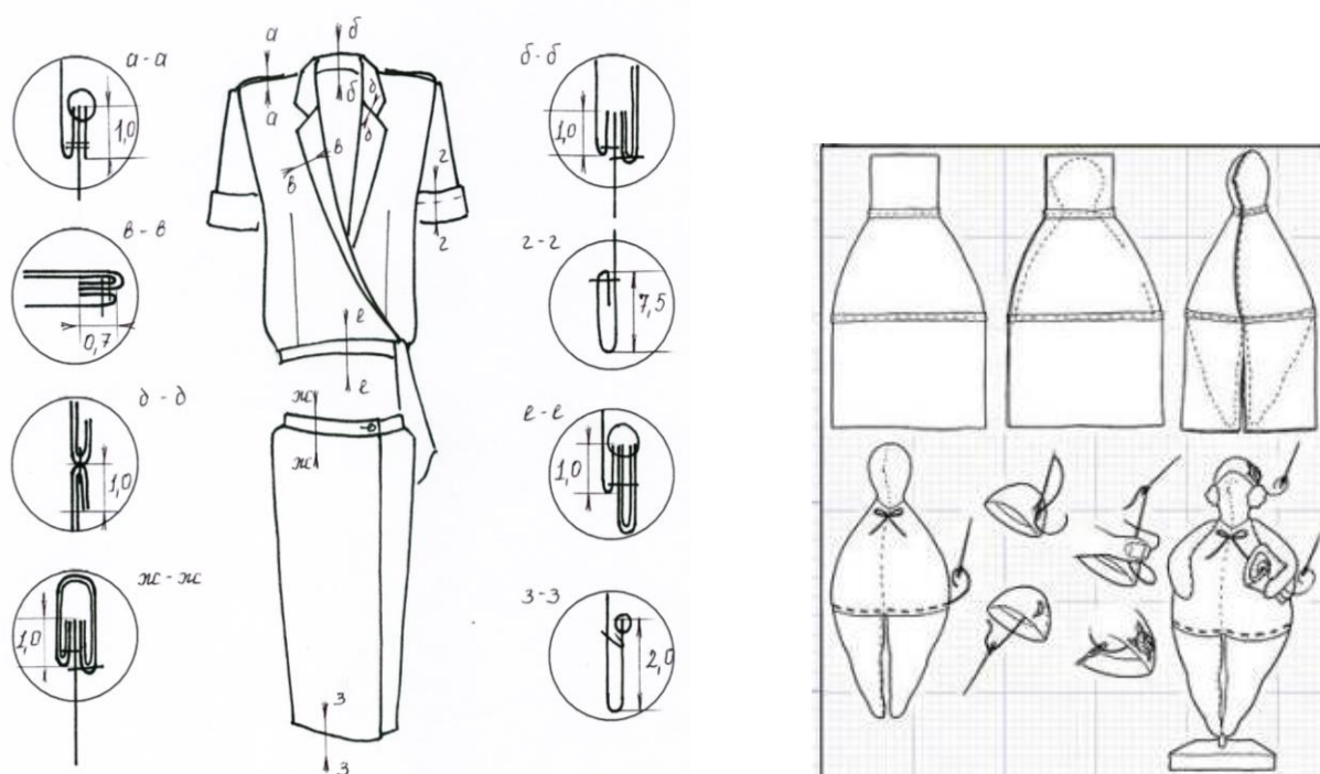
Рисунок 23. Схема обработки основных узлов изделий
