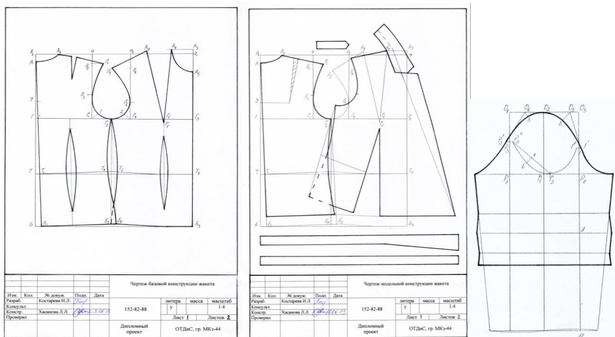
Рисунок 17. Пример оформления чертежей базовой и модельной конструкции
