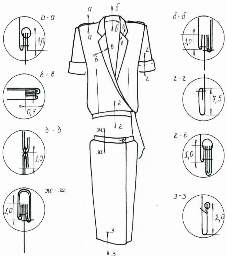
Рисунок 18. Схема обработки основных узлов изделий
